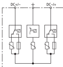
Kapcsolási rajz DG YPV SCI 1000
